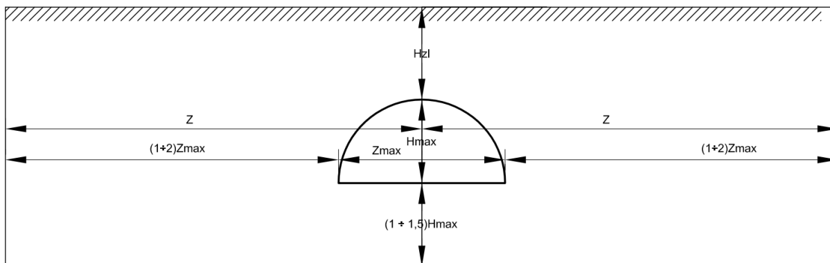
Rysunek 26 Zasięg rozpoznania masywu skalnego w otoczeniu tunelu ( Z = (1,5 \div 2,5)Z_{max} ) - STEŚ-R II Etap oraz KP
