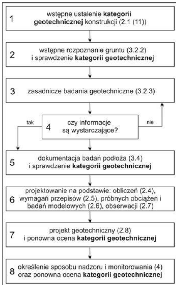
Rysunek 18 Schemat ustalania kategorii geotechnicznej obiektu budowlanego (Majer E., Sokołowska M., Frankowski Z. i in., 2018, Frank et.al., 2004)
