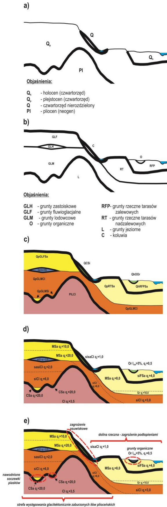
Rysunek 43 Zasady wydzielenia warstw gruntów i skał. a - kompleksy stratygraficzne, b - serie genetyczne, c - warstwy litologiczne, d - warstwy geologiczno-inżynierskie, e - strefy zagrożeń
