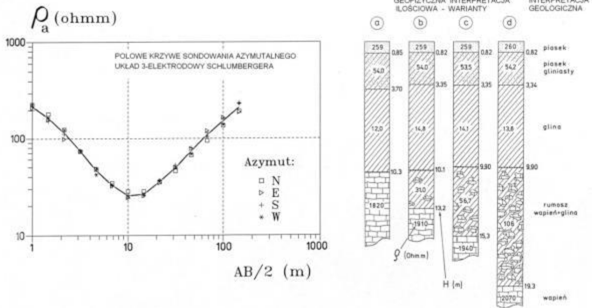
Rysunek 39 Przykład wariantowej interpretacji geofizyczno-geologicznej sondowania elektrooporowego azymutalnego (rozszerzony wariant sondowania krzyżowego)
